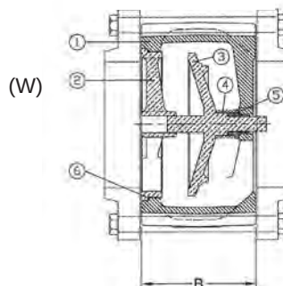
W-910-W-LF/W-960-W-LF Wafer
