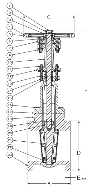
F-617-ON
