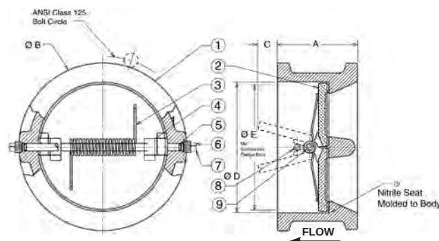
W-920-W-LF Wafer
