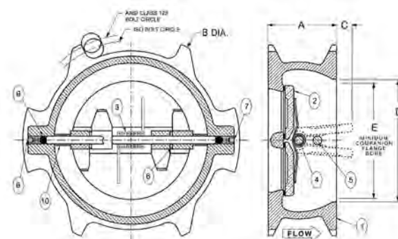
W-920-W-LF Wafer
