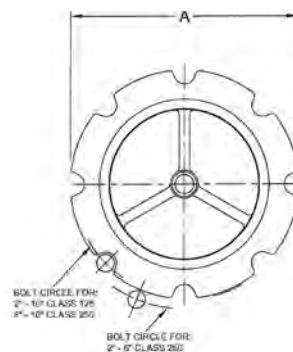
W-910-B-LF/W-960-B-LF Wafer
