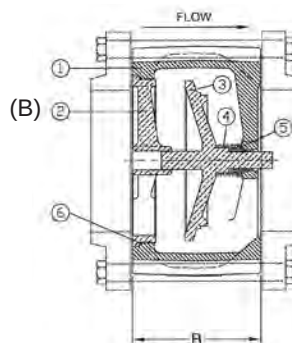
W-910-B-LF/W-960-B-LF Wafer
