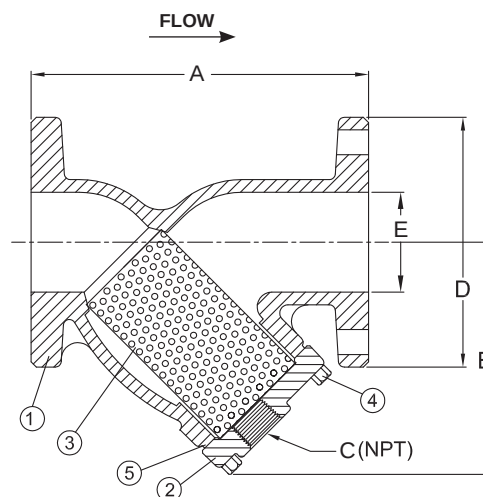
F-721-A Flanged
