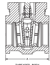
T-617-ON
