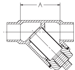
S-221/222-A Solder
